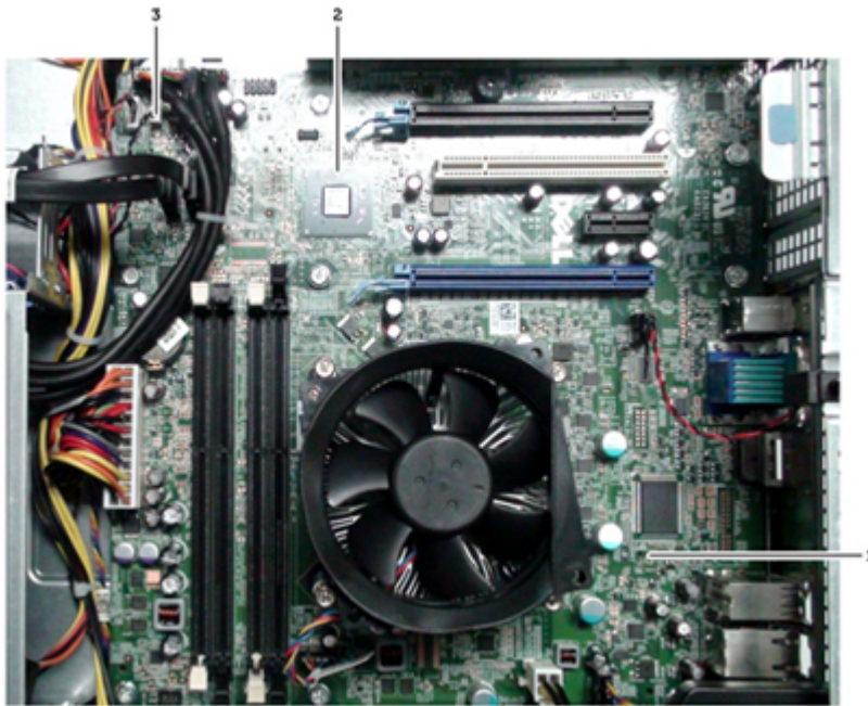
図 2. サーマルセンサーとヒートシンクを備えたシステム基板を取り外した図
